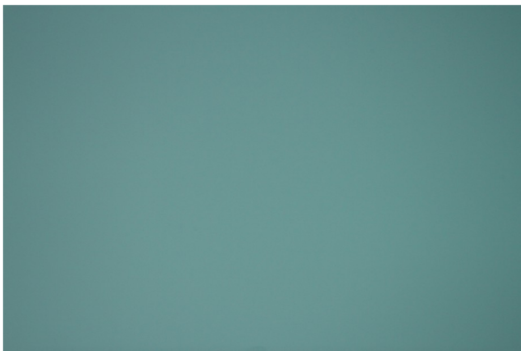
Figura 1: esempio di flat frame acquisito con una DSLR modello Canon EOS 400D modificata Baader.
